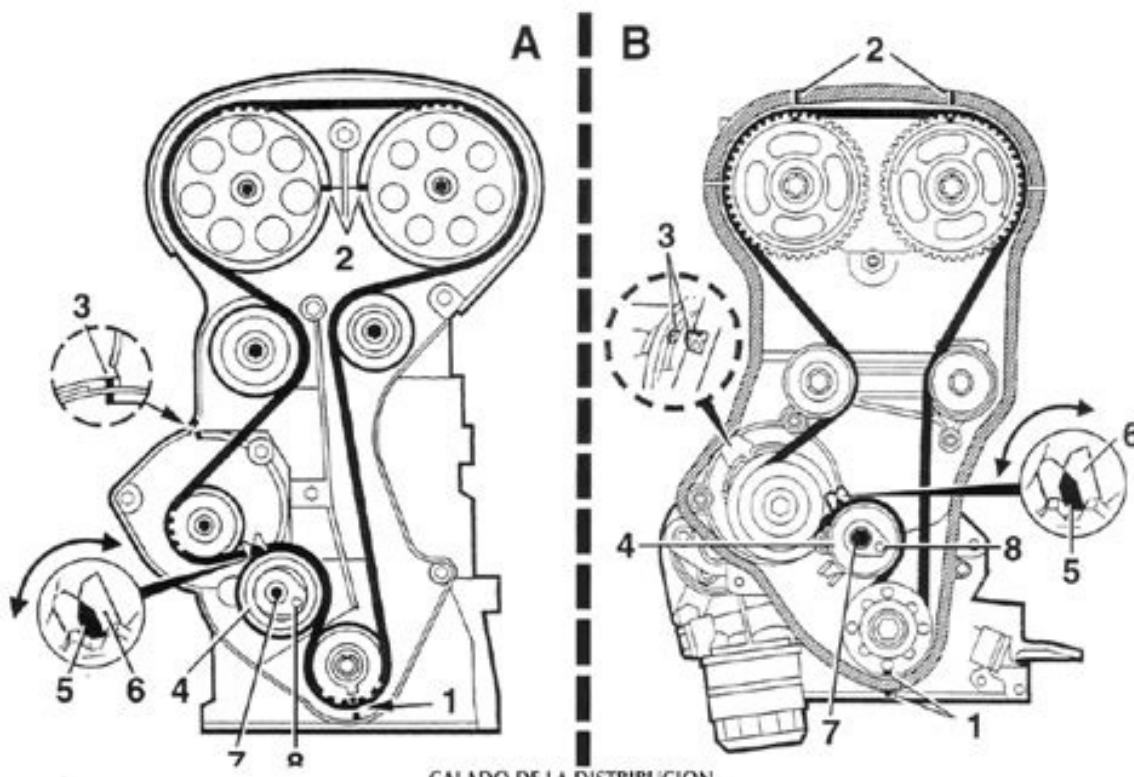
A. Motor 1.6 - 8. Motores 1.8 y 2.0 - 1. Marca de rueda dentada de cigüeñal - 2. Marcas de ruedas dentadas de ejes de levas - 3. Marca de bomba de agua - 4. Rodillo tensor - 5. Indicador de rodillo tensor - 6. Muesca de rodillo tensor - 7. Fijación del rodillo tensor - 8. Hueco hexagonal de reglaje.
